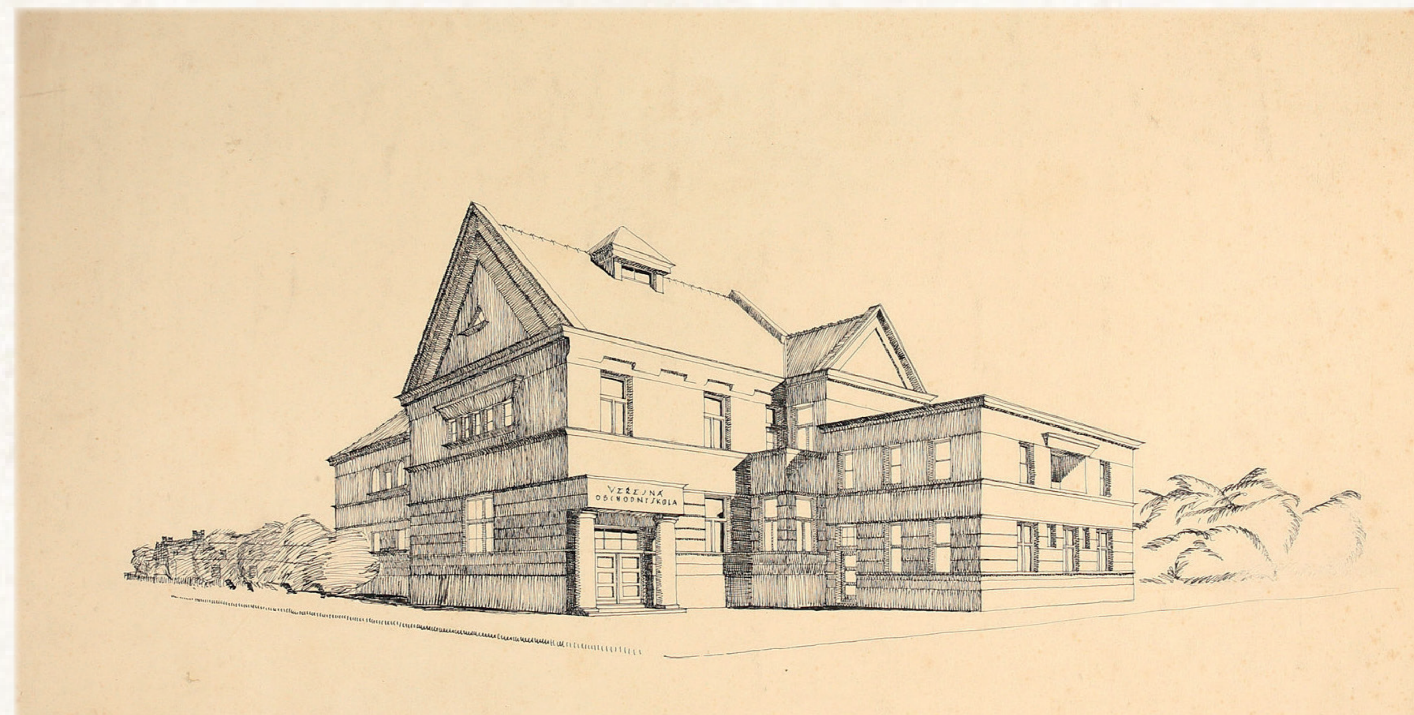
Veřejná obchodní škola, druhý soutěžní návrh Ing. arch. Č. Musila, perspektivní pohled, 1929 (Státní oblastní archiv v Zámrsku – Státní okresní archiv Jičín, Fond Musil Čeněk, projekt č. 164, Obchodní škola v Jičíně, 1929)
